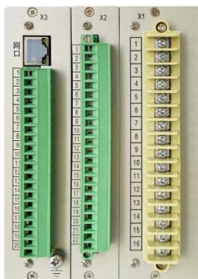
背视图
