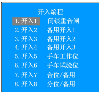
图 5.4 -16 开入编辑设置画面图
