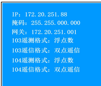
图 5.4 -15 以太网设置画面图
