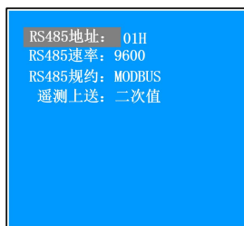
图 5.5-12 RS485 设置画面图
