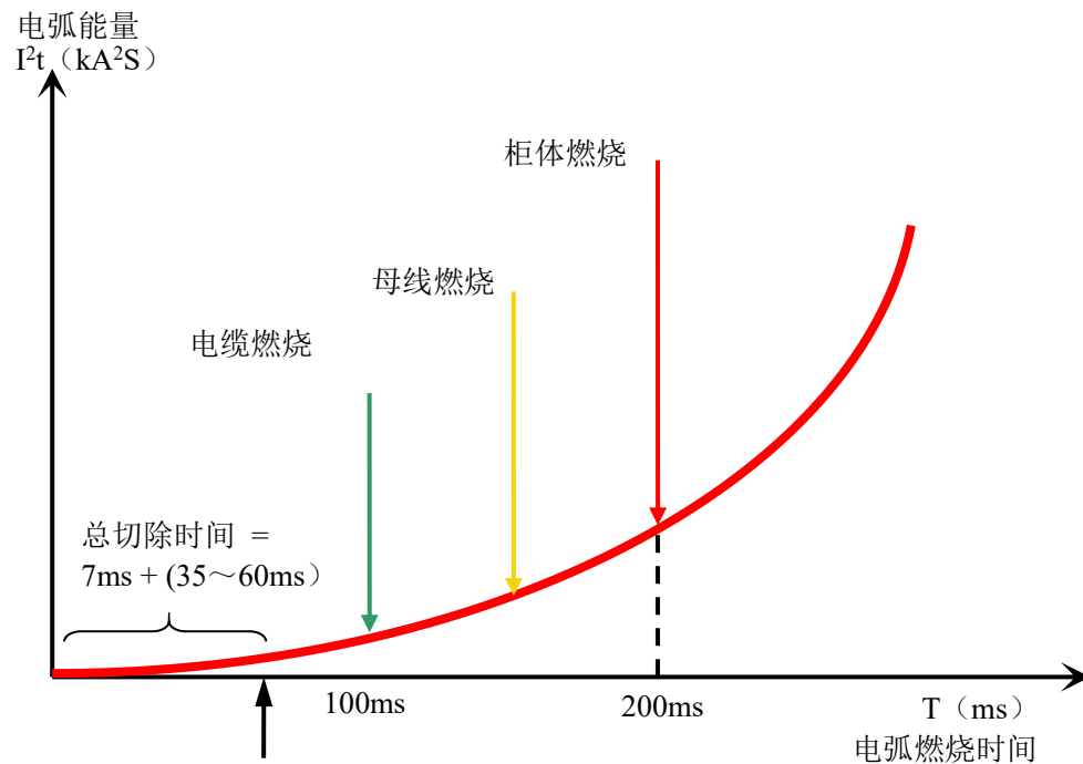
电弧光危害示意图
