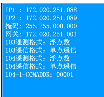
图 5.4 -15 以太网设置画面图
