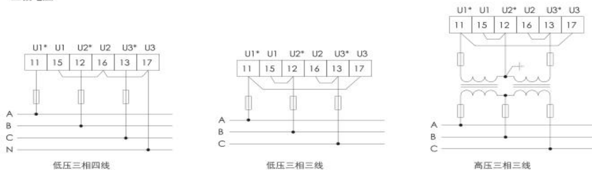
07 外形电压表输入信号接线图
