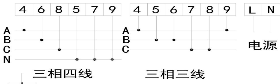
不带辅助功能且是交流 220V 电源的 09 外形电压表接线图
