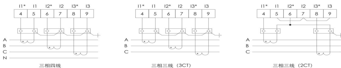
三相电流
