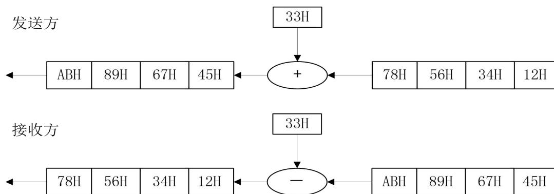
图 2 传输次序图
