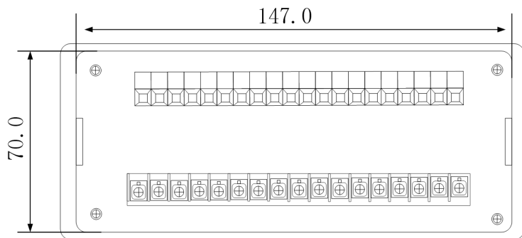
背板图
